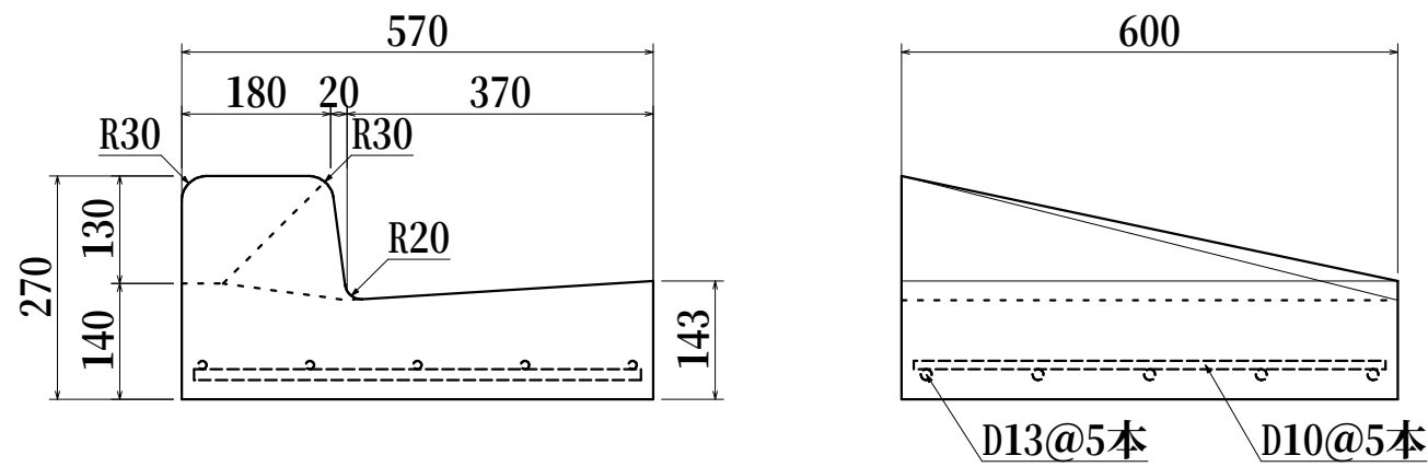
千葉県土木型570 柏市 摺付け部 約126kg
