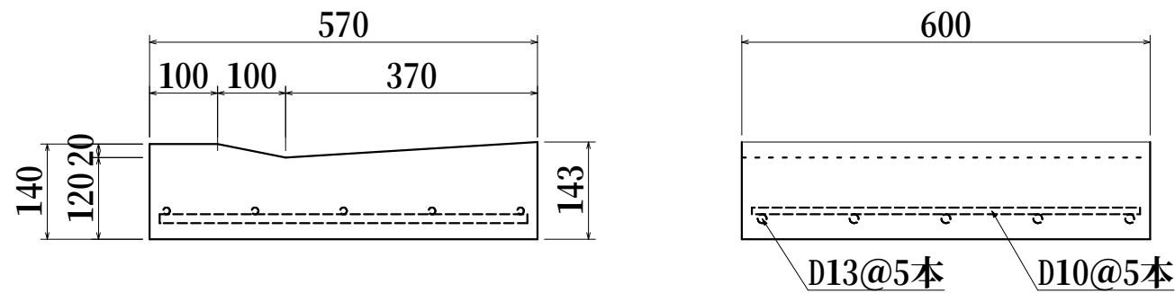
千葉県土木型570 柏市 平坦部0/20 約108kg
