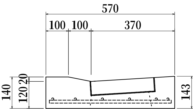
千葉県土木型570 柏市 平0/20 縁塊 約102kg
