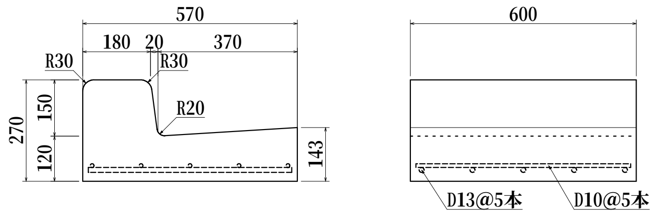
千葉県土木型570 柏市 基本型 約144kg
