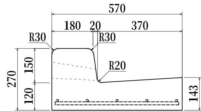
千葉県土木型570 柏市 基本型（水抜き） 約131kg
