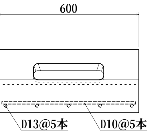
千葉県土木型570 柏市 基本型（水抜き） 約131kg
