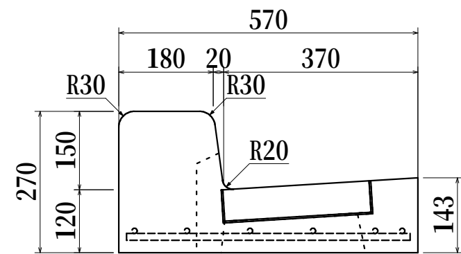
千葉県土木型570 柏市 基本型 縁塊 約132kg
