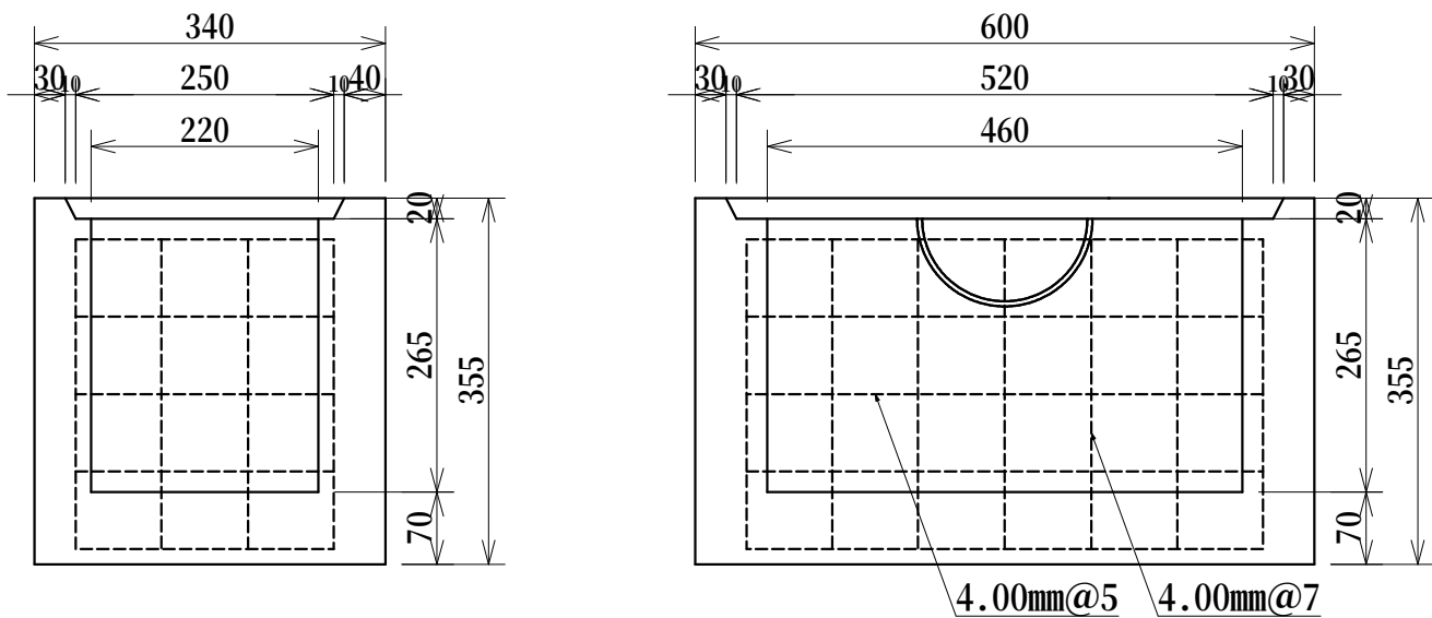
LU街渠 枅用下部側塊 240 (薄、厚兼用) 参考荷重 約102kg
