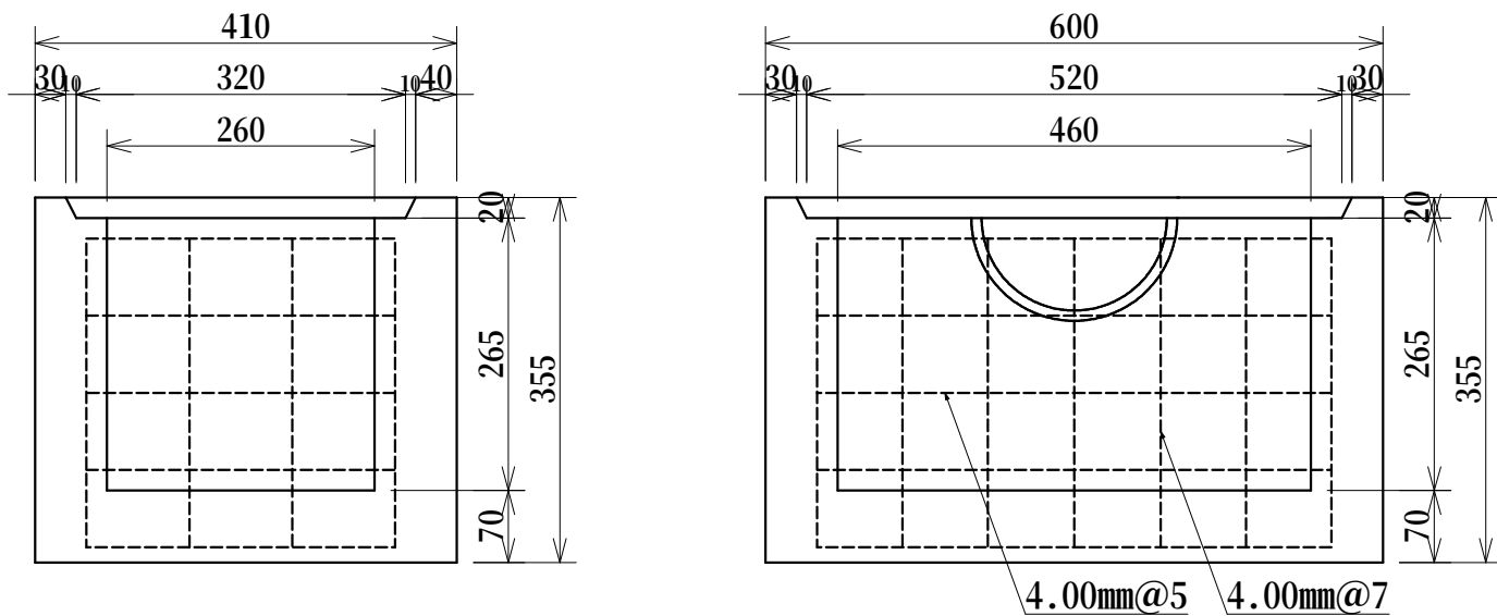
LU街渠 枅用下部側塊 300 (薄、厚兼用) 参考荷重 約126kg
