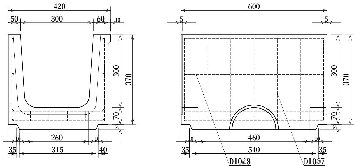
LU街渠 枅用上部側塊 300 (薄、厚兼用) 参考荷重 約79kg
