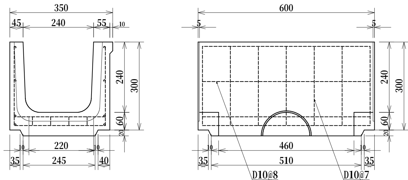
LU街渠 枅用上部側塊 240 (薄、厚兼用) 参考荷重 約54kg
