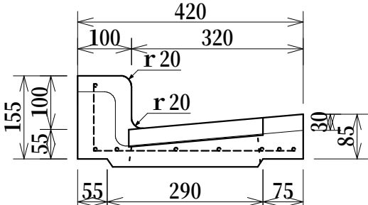
LU街渠300（薄）真物縁塊 参考荷重 約43kg
