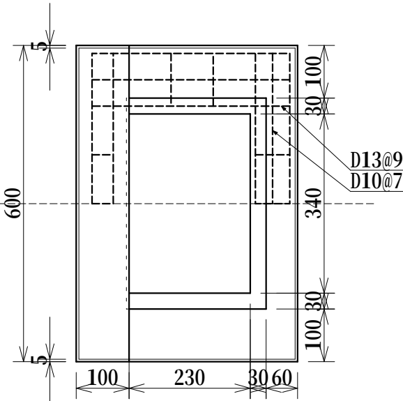
LU街渠300（厚）真物縁塊 参考荷重 約59kg
