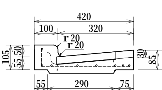
LU街渠300（薄）平5cm縁塊 参考荷重 約36kg
