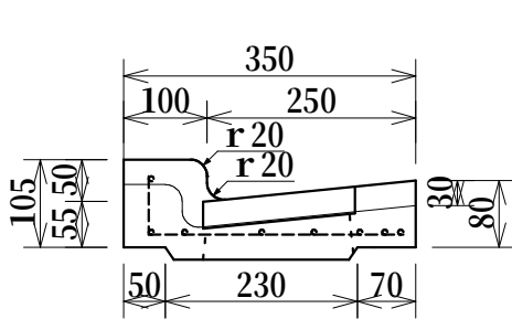
LU街渠240（薄）平5cm縁塊 参考荷重 約32kg
