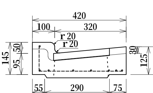
LU街渠300（厚）平5cm縁塊 参考荷重 約52kg
