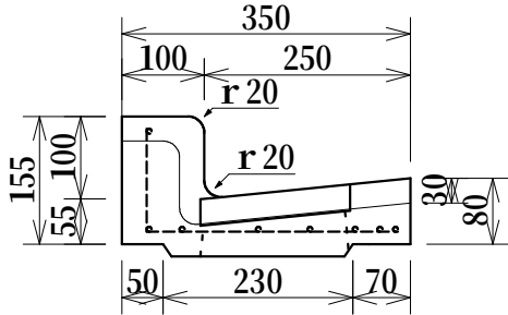
LU街渠240（薄）真物縁塊 参考荷重 約39kg
