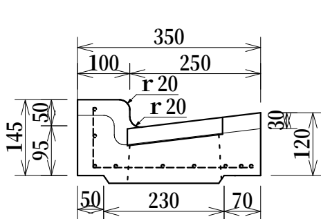
LU街渠240（厚）平5cm縁塊 参考荷重 約45kg
