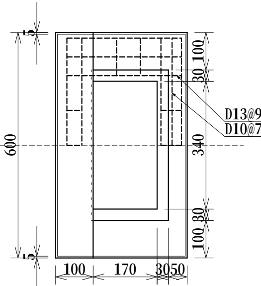
LU街渠240（厚）真物縁塊 参考荷重 約52kg
