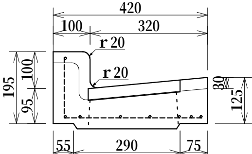
LU街渠300（厚）真物縁塊 参考荷重 約59kg
