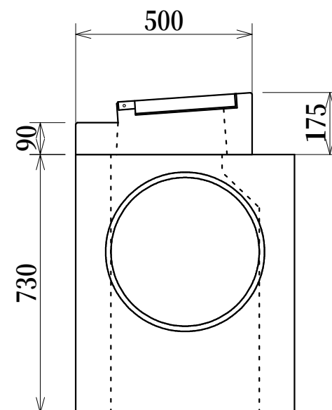
性能規定型雨水柵タイプ2 縁塊 500×600×90/175
