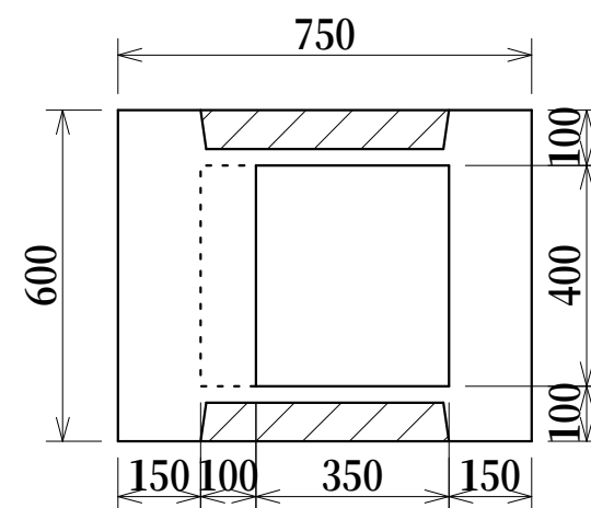
旧L0柵タイプ1
