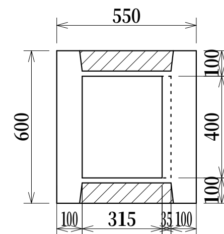
L0柵タイプ4
