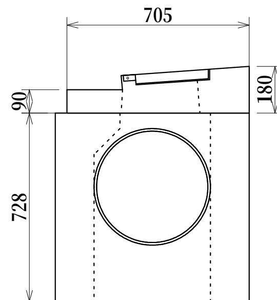
性能規定型雨水柵タイプ1-B 縁塊 705×600×90/180
