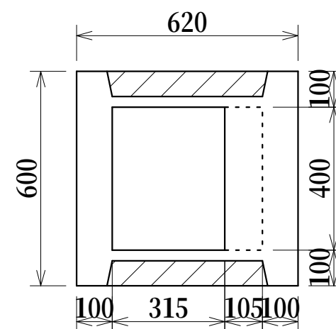
L0柵タイプ3
