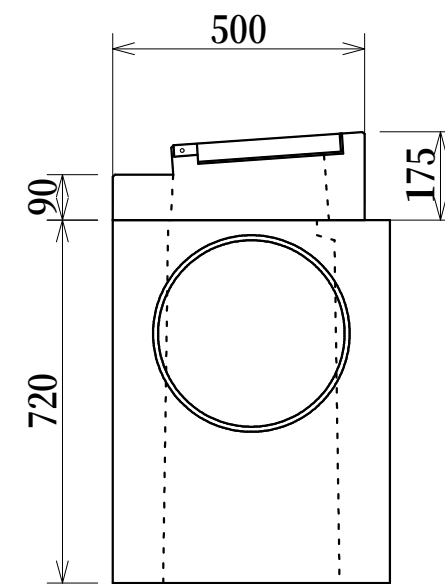
性能規定型雨水柵タイプ2 縁塊 500×600×90/175
