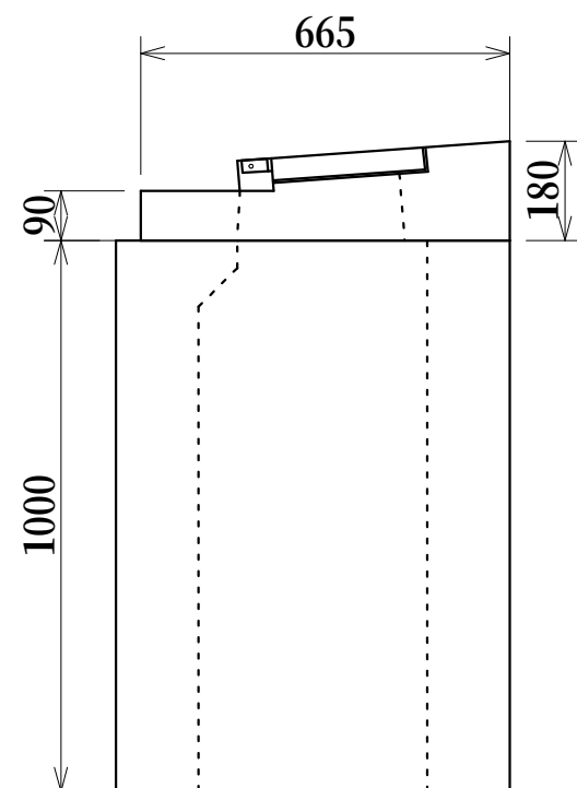
性能規定型雨水柵タイプ1-A 縁塊 665×600×90/180
