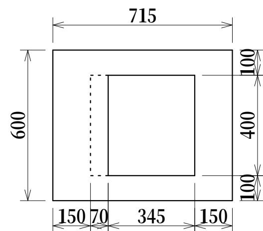
新L0柵タイプ1
