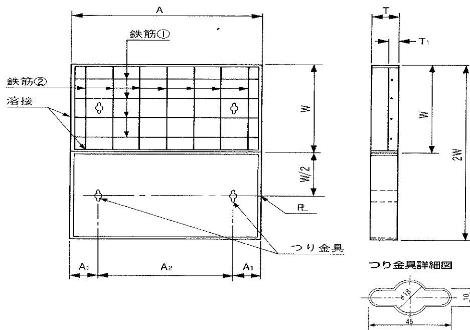
寸法表
