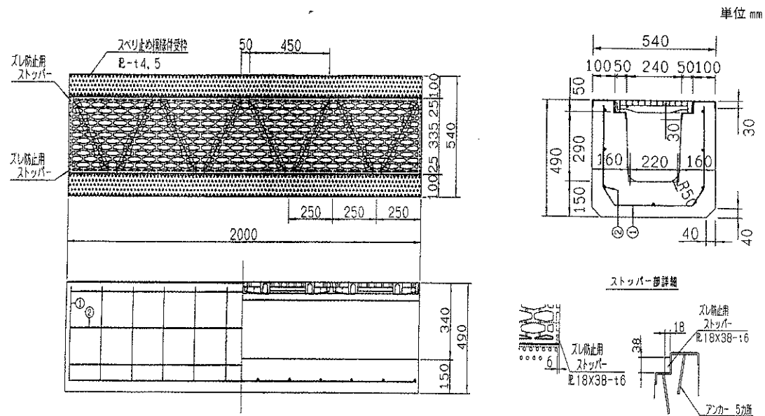
配筋
