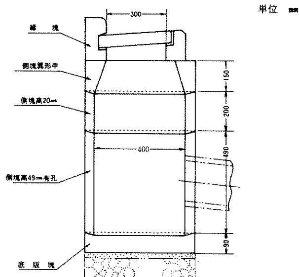
(例) L形用集水柵300
