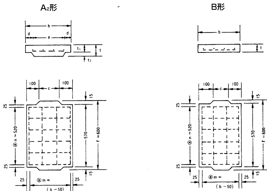
ふたの種類
