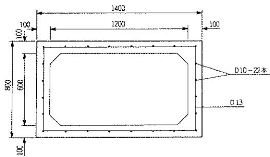
側塊1号
