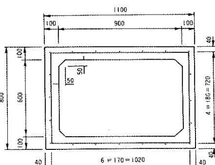
側塊 3号
