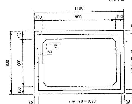
側塊 5号
