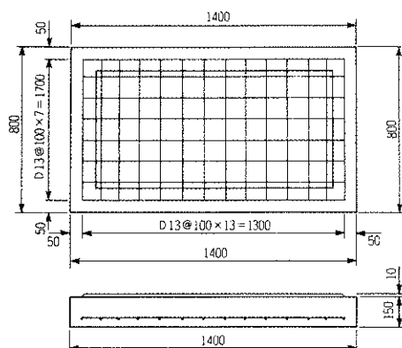
底板塊
