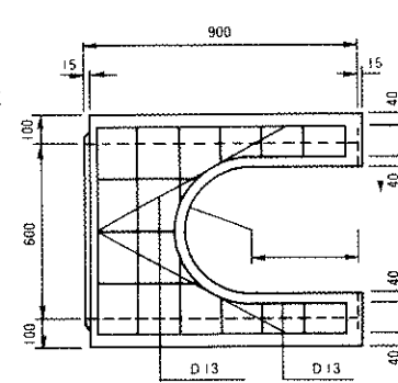
孔明部補強図
