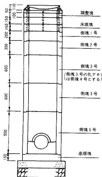
横断面図
