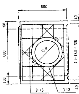
孔明部補強図
