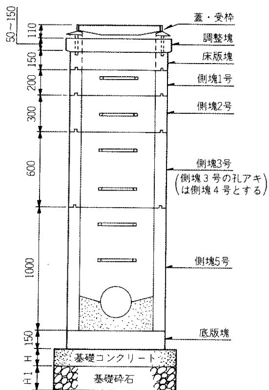
横断面図
