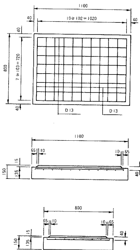
底版塊
