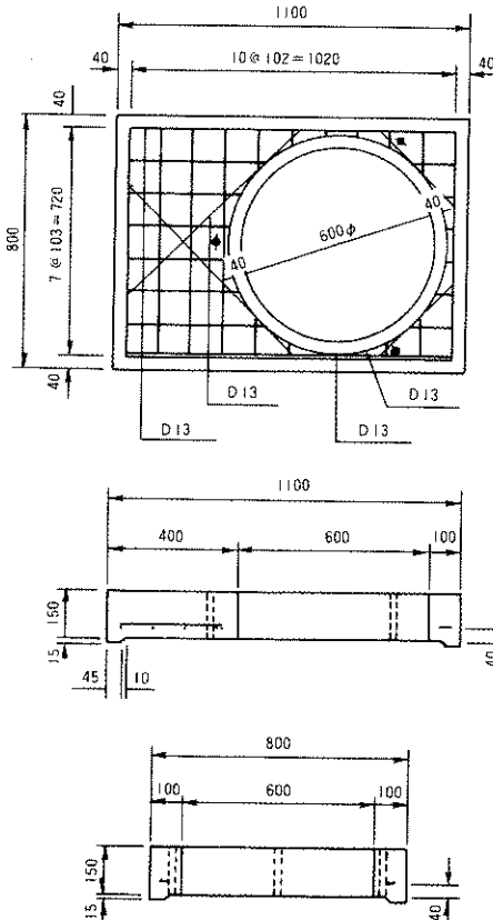
床版塊
