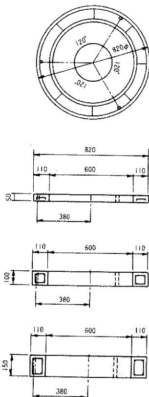
調整塊
