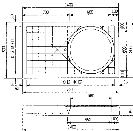
床版塊
