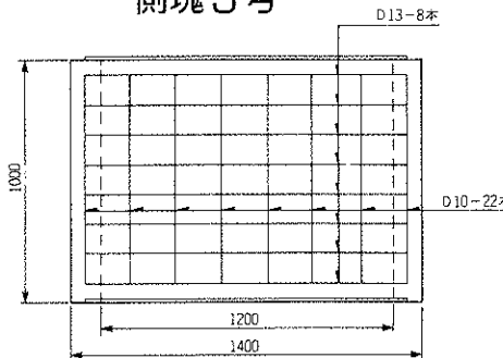
側塊5号
