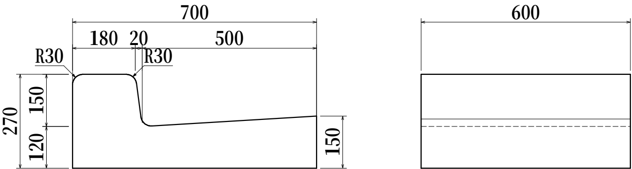
国交省 L形Ⅱ型 柏市型 基本型
