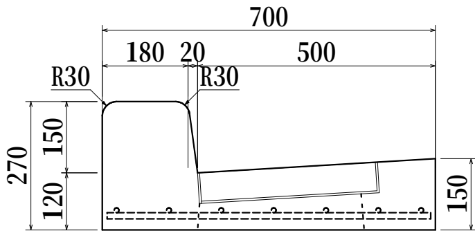
国交省 L形縁塊 柏市型 基本型
