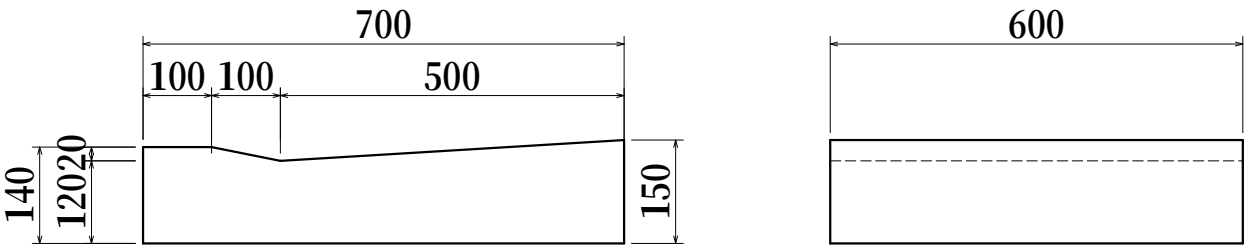
国交省 L形Ⅱ型 柏市型 平坦部0/20
