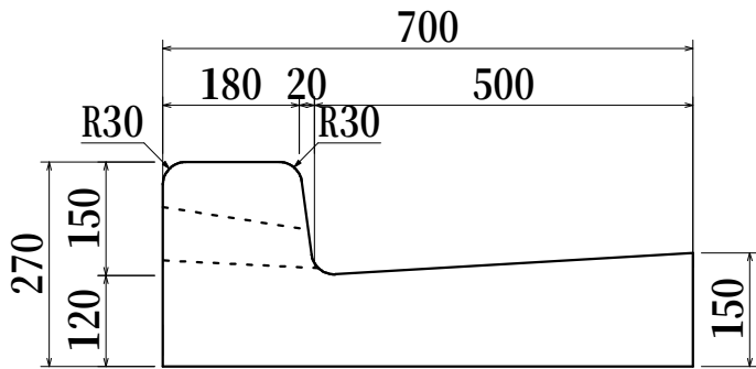
国交省 L形Ⅱ型 柏市型 基本型（水抜き）
