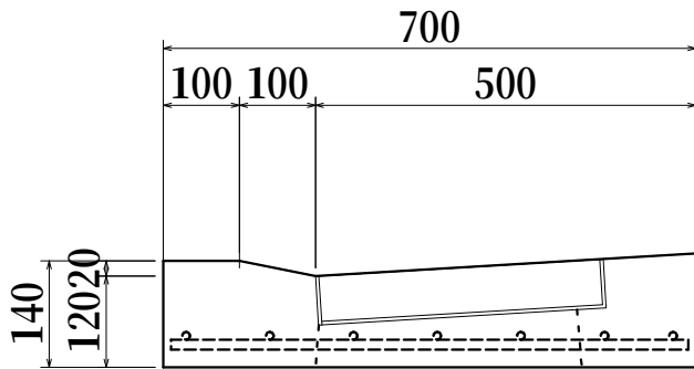
国交省 L形縁塊 柏市型 平坦部0/20
