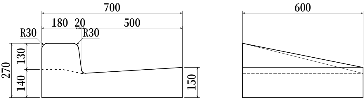
国交省 L形Ⅱ型 柏市型 摺付け部
