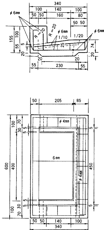
240用 縁塊
