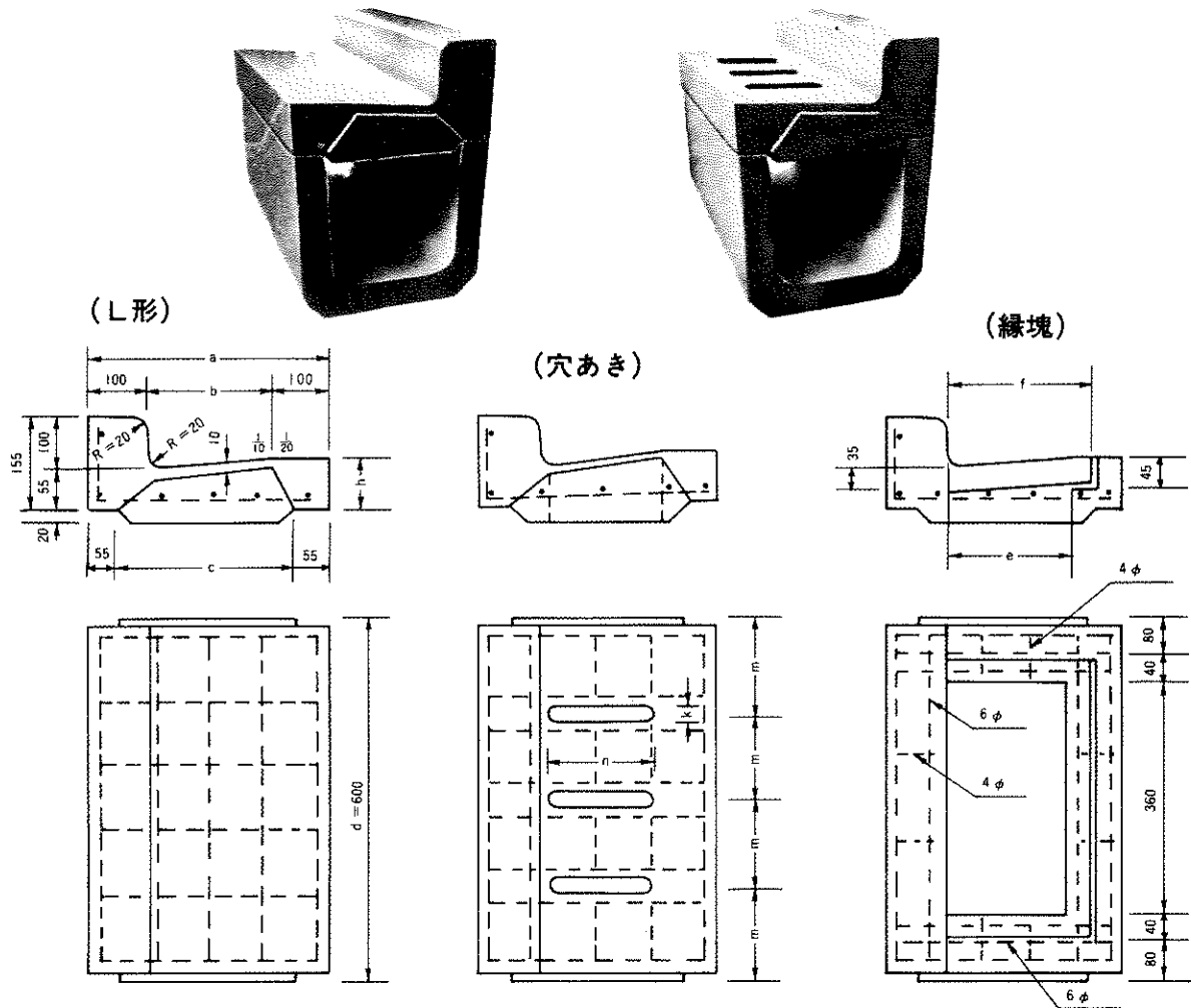
寸法および鉄筋
