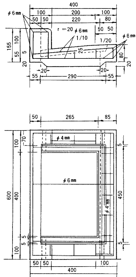
ふた（鋳鉄製）
