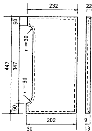
ふた（鋳鉄製）
