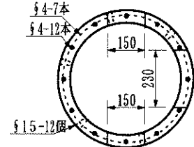
浸透側塊 (有孔)
