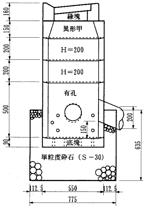
雨水浸透枡構造図
