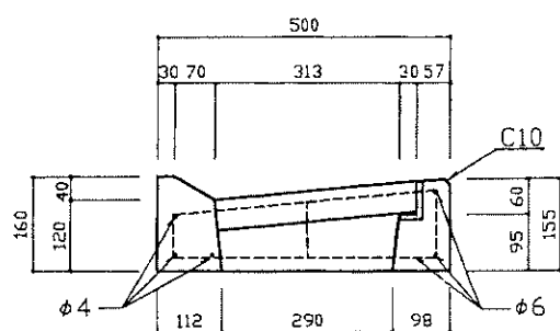
縁塊
