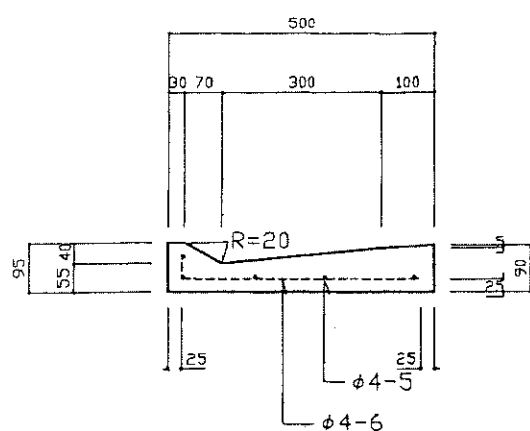
L形
