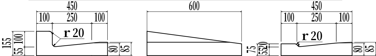
L形側溝 1種250B 真物 から 1種250B 平2cm 落ち 左右 重量 約52kg
