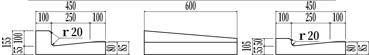
L形側溝 1種250B 真物 から 1種250B 平5cm 落ち 左右 重量 約53kg
