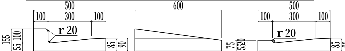
L形側溝 1種300B 真物 から 1種300B 平2cm 落ち 左右 重量 約58kg
