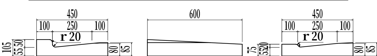
L形側溝 1種250B 平5cm から 1種250B 平2cm 落ち 左右 重量 約47kg
