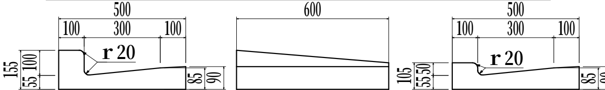
L形側溝 1種300B 真物 から 1種300B 平5cm 落ち 左右 重量 約59kg
