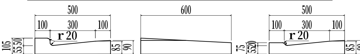
L形側溝 1種300B 平5cm から 1種300B 平2cm 落ち 左右 重量 約56kg
