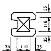
断面 A—A
