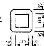
断面 B—B
