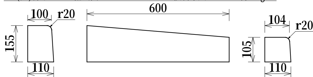
(旧)都市基盤整備公団型ブロックE100A 1段斜乗入 重量 約20kg
