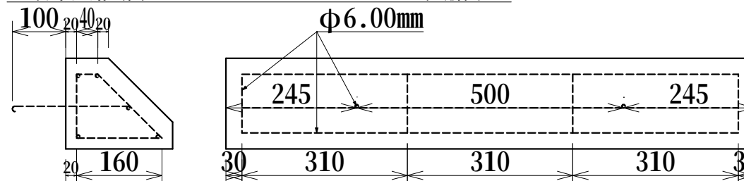
日本道路公団型マンタブルブロック L=990 配筋図
