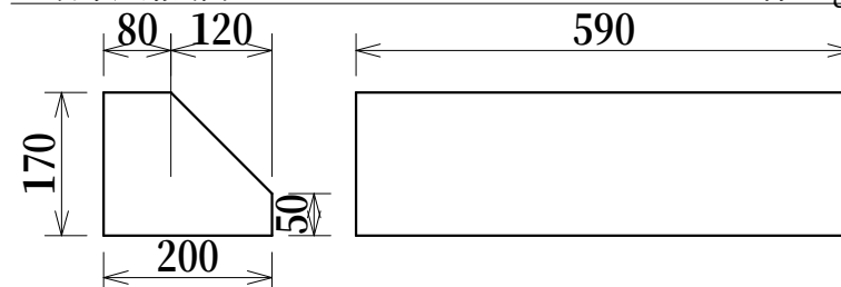
日本道路公団型マンタブルブロック L=590 重量 約38kg
