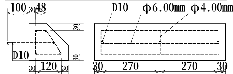
首都高速道路公団型マンタブルブロック L=600 配筋図
