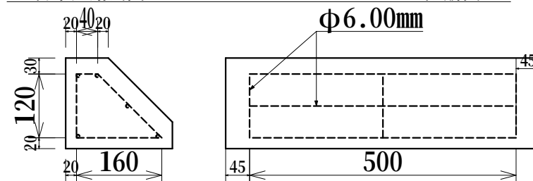
日本道路公団型マンタブルブロック L=590 配筋図
