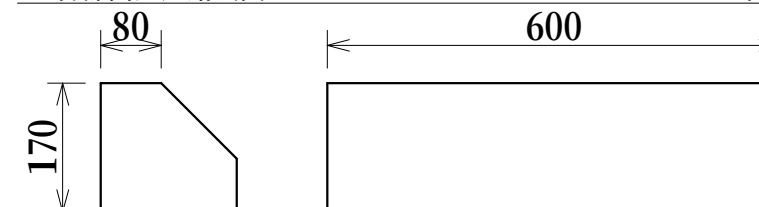
首都高速道路公団型マンタブルブロック L=600 重量 約37kg
