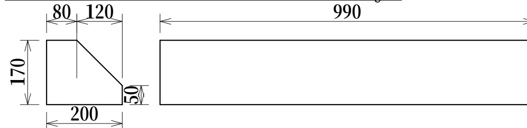
日本道路公団型マンタブルブロック L=990 重量 約63kg
