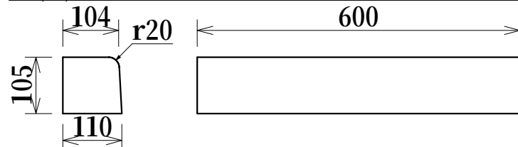
(旧)都市基盤整備公団型ブロックE100A 乗入 重量 約17kg
