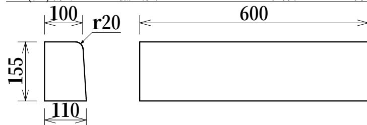
(旧)都市基盤整備公団型ブロックE100A 真物 重量 約23kg
