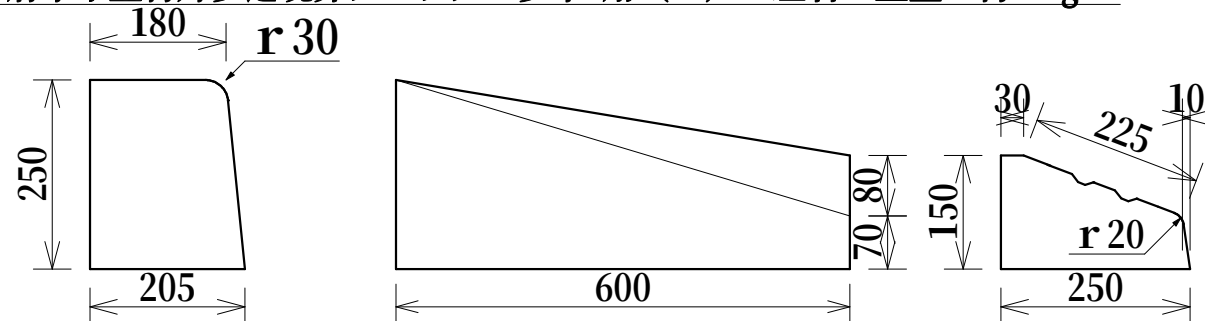
府中市型特殊歩道境界ブロック 歩車B用 (A4) 左右 重量 約52kg
