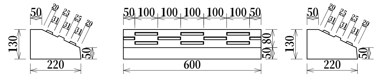
改良江戸川型特殊歩道境界ブロック 乗入 重量 約32kg
