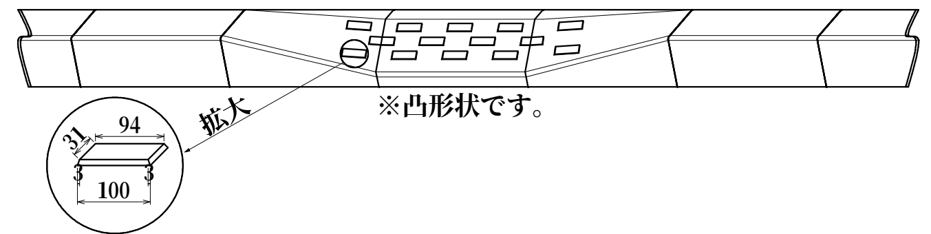
改良江戸川型特殊歩道境界ブロック 斜 左右 重量 約39kg
