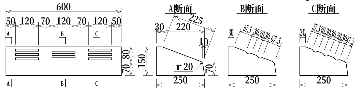
府中市型特殊歩道境界ブロック 歩車A・B兼用乗入 (B3) 重量 約40kg
