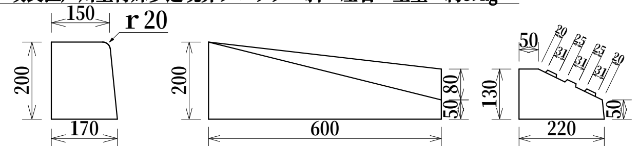
改良江戸川型特殊歩道境界ブロック 斜 左右 重量 約39kg
