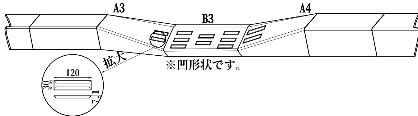
府中市型特殊歩道境界ブロック 歩車A用 (A3) 左右 重量 約42kg
