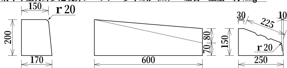
府中市型特殊歩道境界ブロック 歩車A用 (A3) 左右 重量 約42kg
