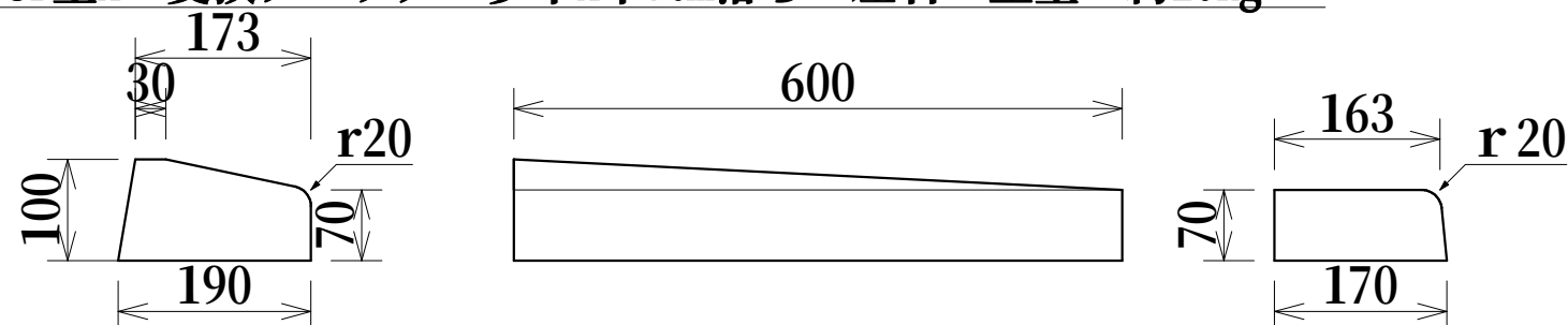
SF型A 変換ブロック 歩車A平7cm落ち 左右 重量 約20kg
