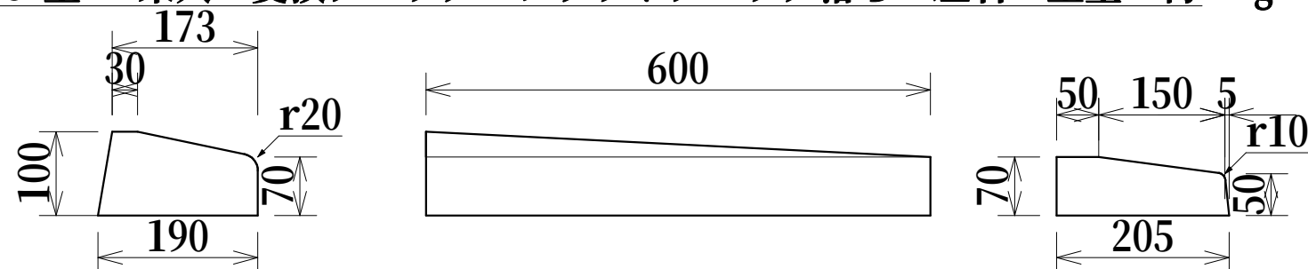
SF型A 乗入 変換ブロック フラットブロック落ち 左右 重量 約21kg
