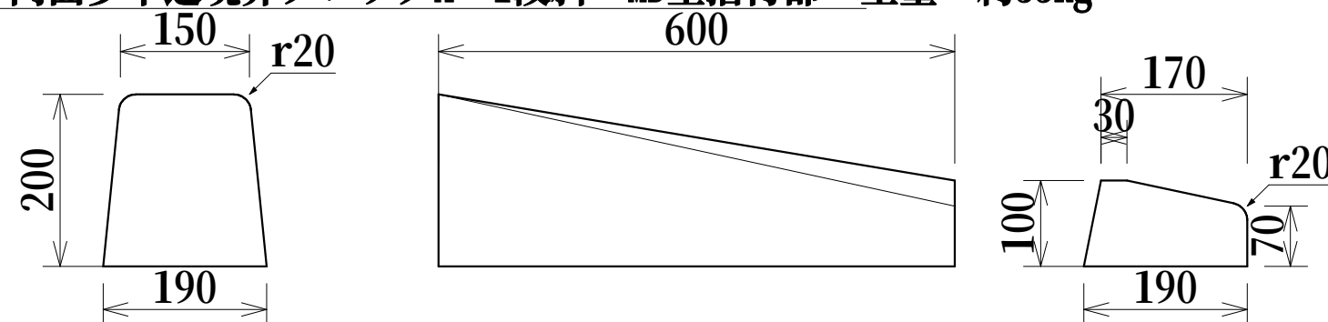
両面歩車道境界ブロックA 1段斜 MD型摺付部 重量 約35kg
