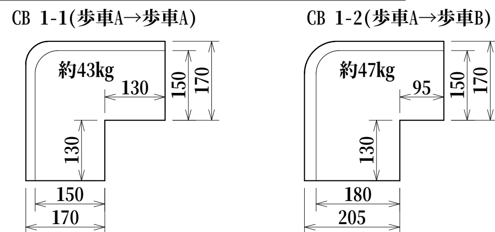
歩車道境界ブロック コーナー部 (外R)
