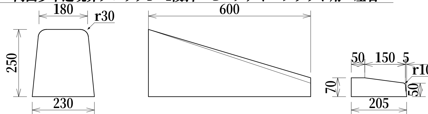
両面歩車道境界ブロックB 1段斜 セーフティ・フラット用 左右
