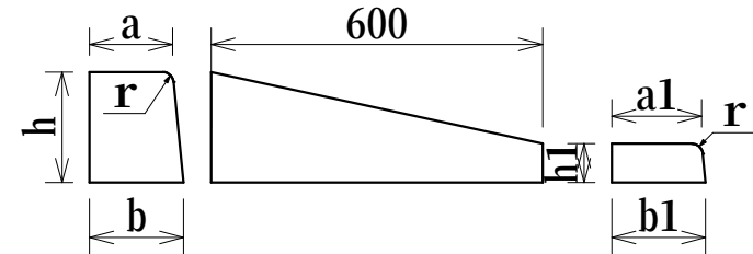
歩車道境界ブロック 2段斜（左右）
