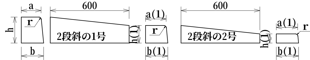
歩車道境界ブロック 3段斜（左右）
