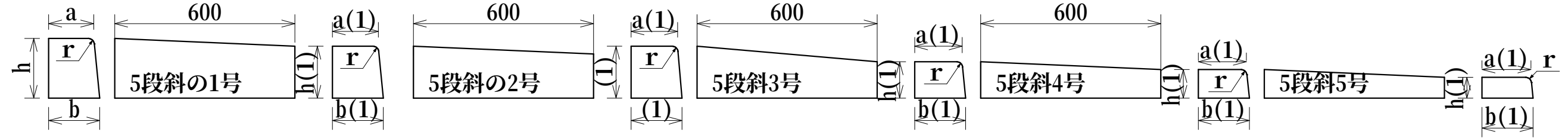
歩車道境界ブロック 5段斜（左右）
