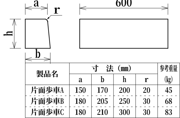
歩車道境界ブロック 基本（真物）
