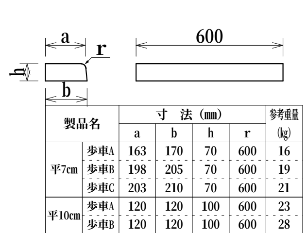
歩車道境界ブロック 平7cm、平10cm
