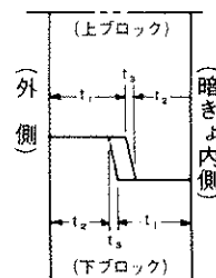
上下組合せ部 詳細図
