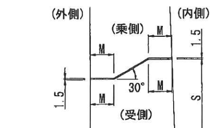
ジョイントテーパー部詳細図
