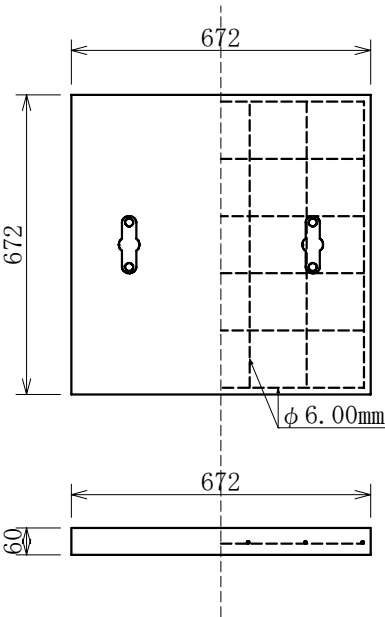
汚水蓋 重量 約56kg
