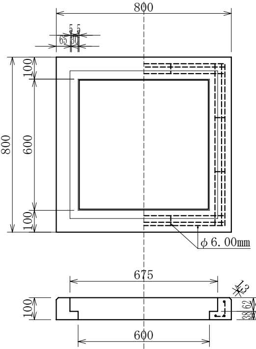
縁塊 重量 約57kg
