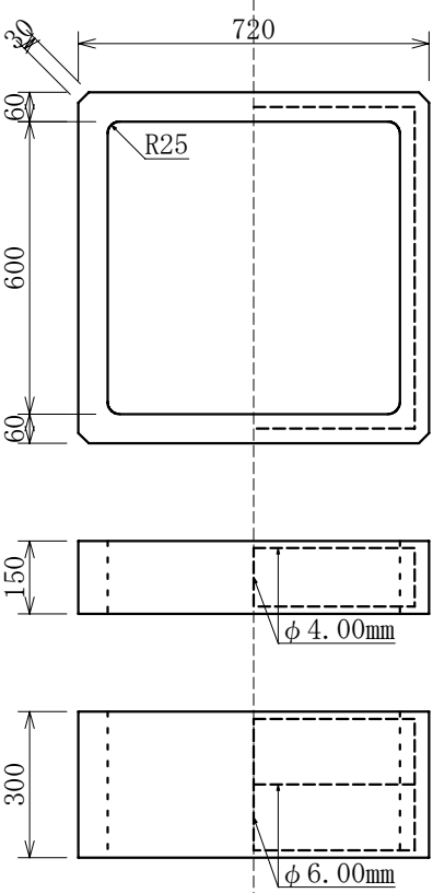
側塊 H=300 重量 約116kg
