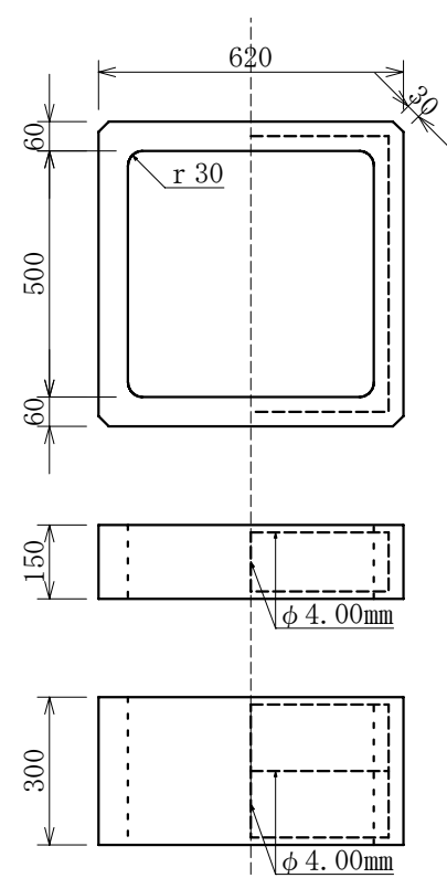
側塊 H=300 重量 約100kg
