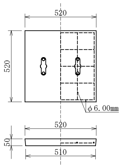
汚水蓋 重量 約33kg
