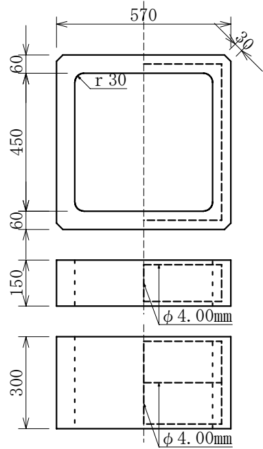
側塊 H=300 重量 約85kg
