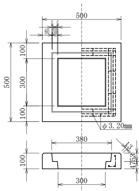
縁塊 重量 約32kg
