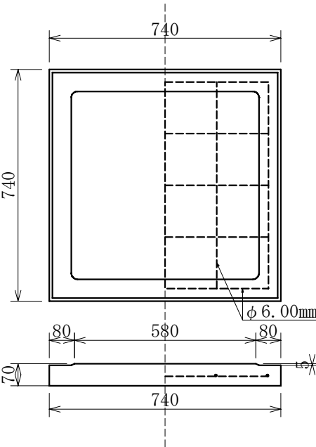
底塊 重量 約94kg
