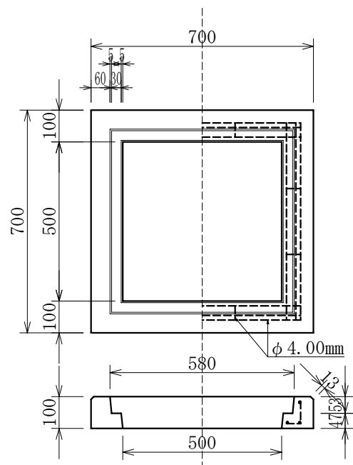
縁塊 重量 約50kg
