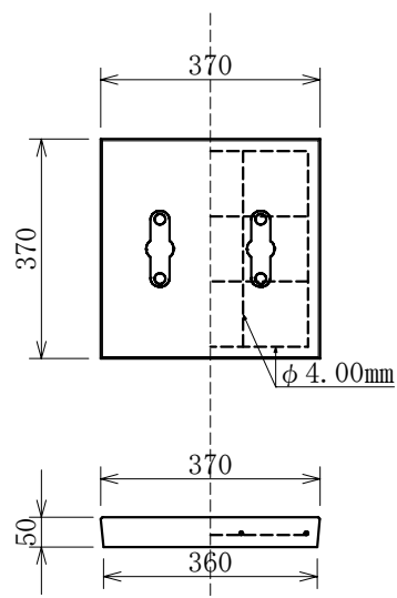
汚水蓋 重量 約17kg
