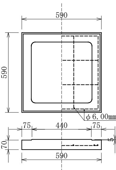
底塊 重量 約60kg
