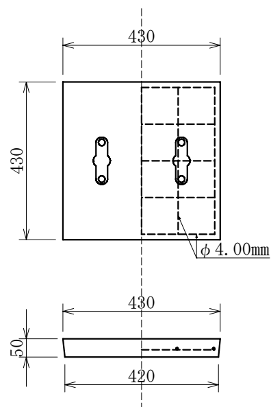
汚水蓋 重量 約23kg
