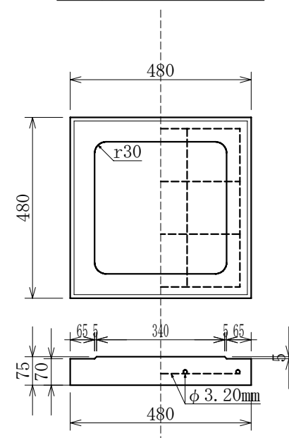
底版 重量 約43kg
