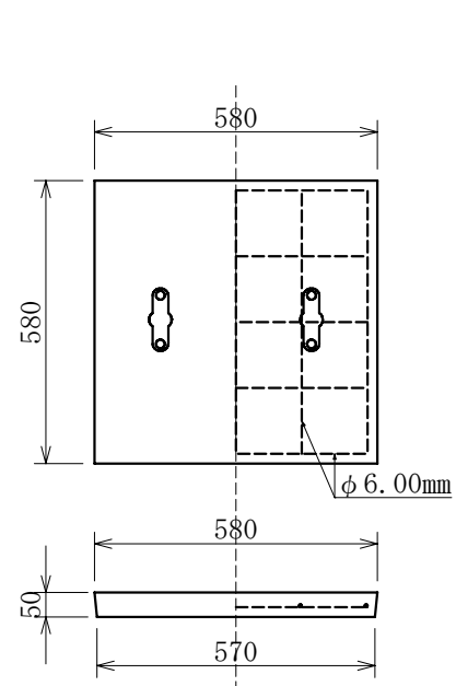
汚水蓋 重量 約40kg
