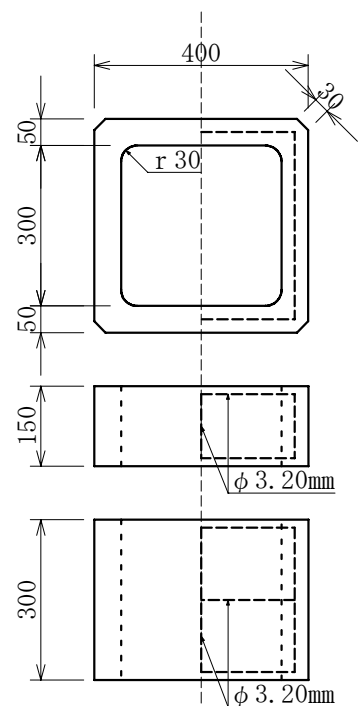
側塊 H=150 重量 約25kg
