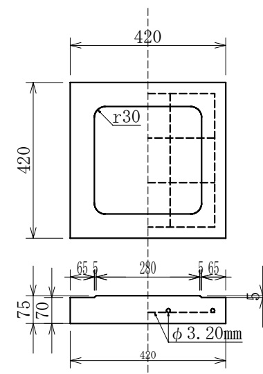
底版 重量 約33kg
