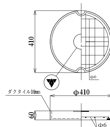
蓋 参考重量 24kg
