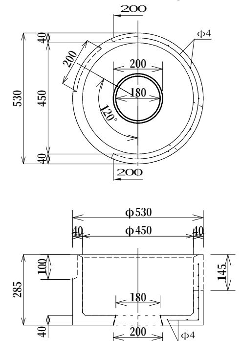
ドロップ底塊 参考重量 50kg
