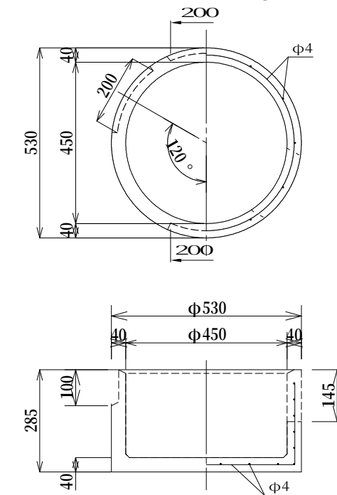
底塊 参考重量 54kg
