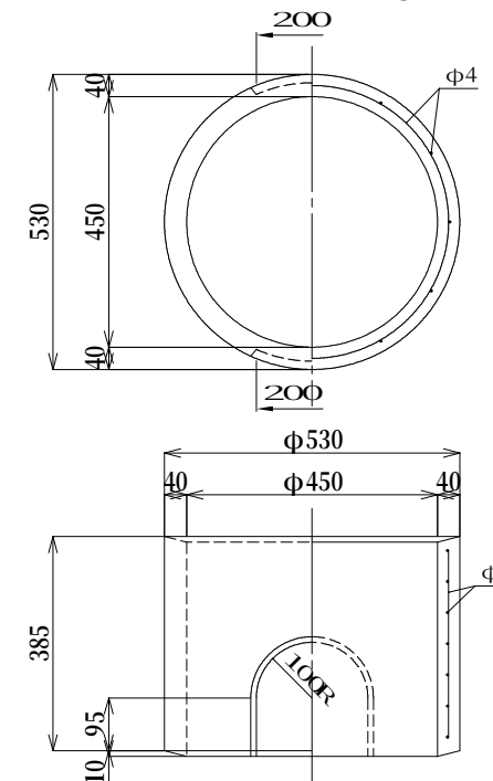
下部側塊 参考重量 52kg
