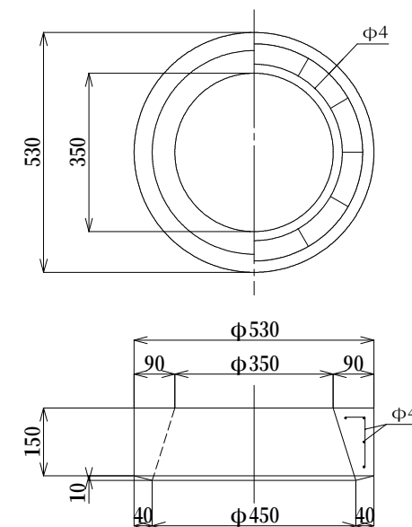
上部隈塊 参考重量 35kg
