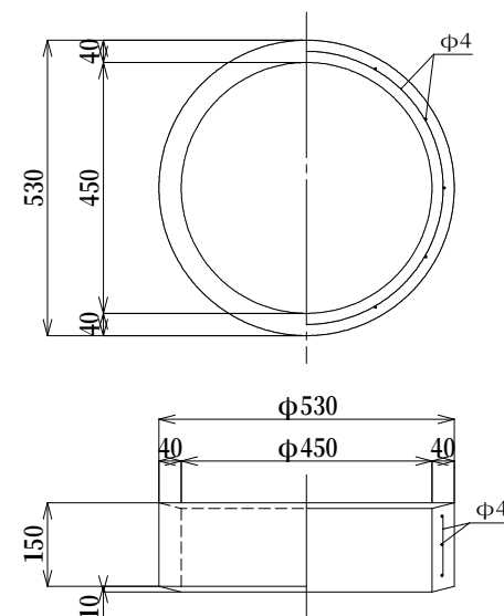
中部側塊 参考重量 22kg
