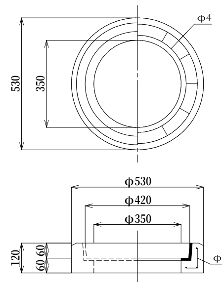
縁塊 参考重量 36kg
