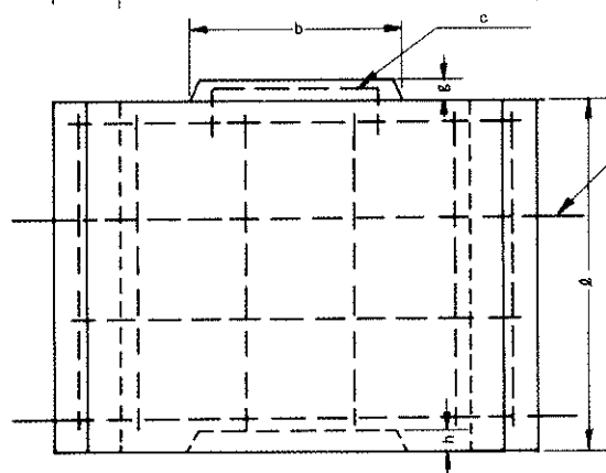
寸法、鉄筋および重量
