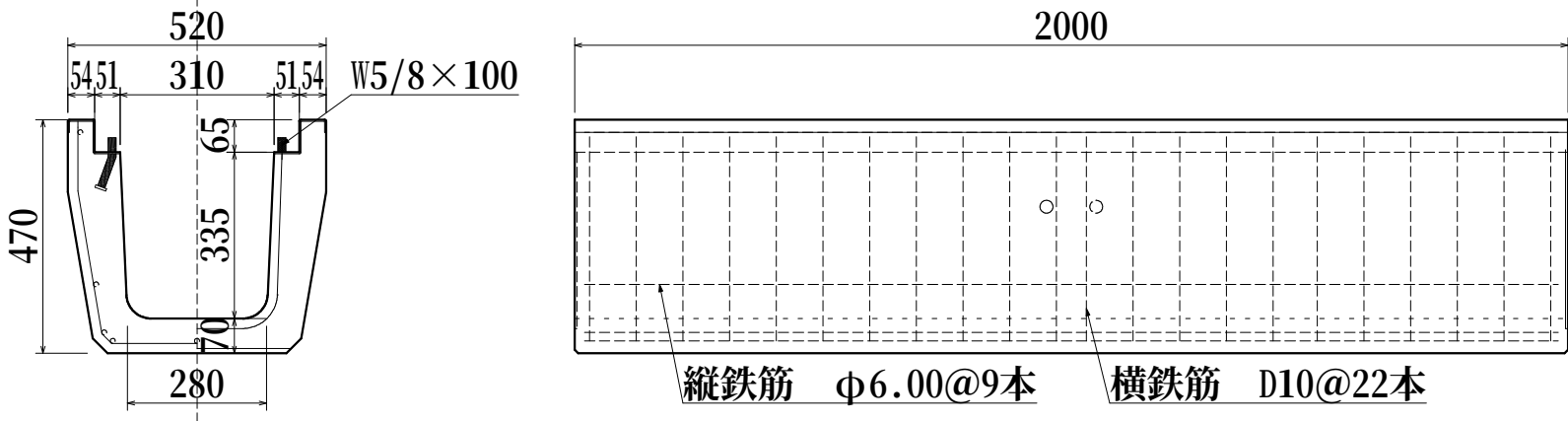
横断側溝（固定式） 300A T-25 約487kg
