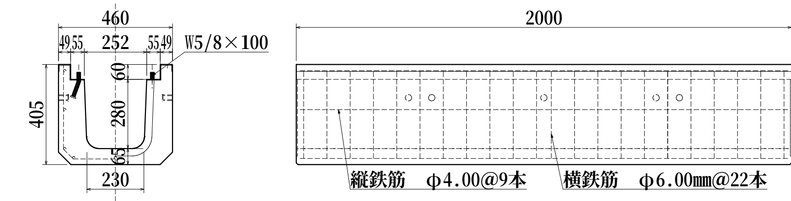
横断側溝（固定式） 250 T-25 約454kg
