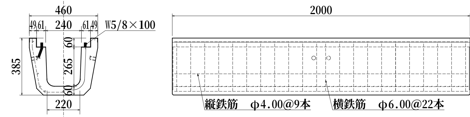
横断側溝（固定式） 240A T-25 約362kg
