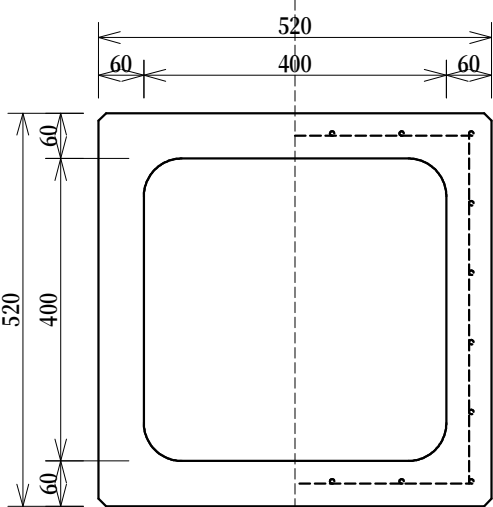
下部側塊 重量 約159kg
