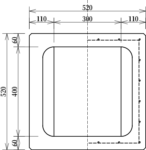
上部側塊 重量 約93kg
