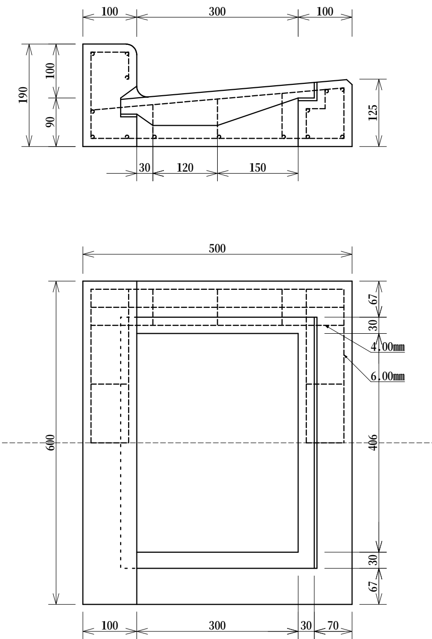
川崎市型雨水枡用真物縁塊 重量 約58kg
