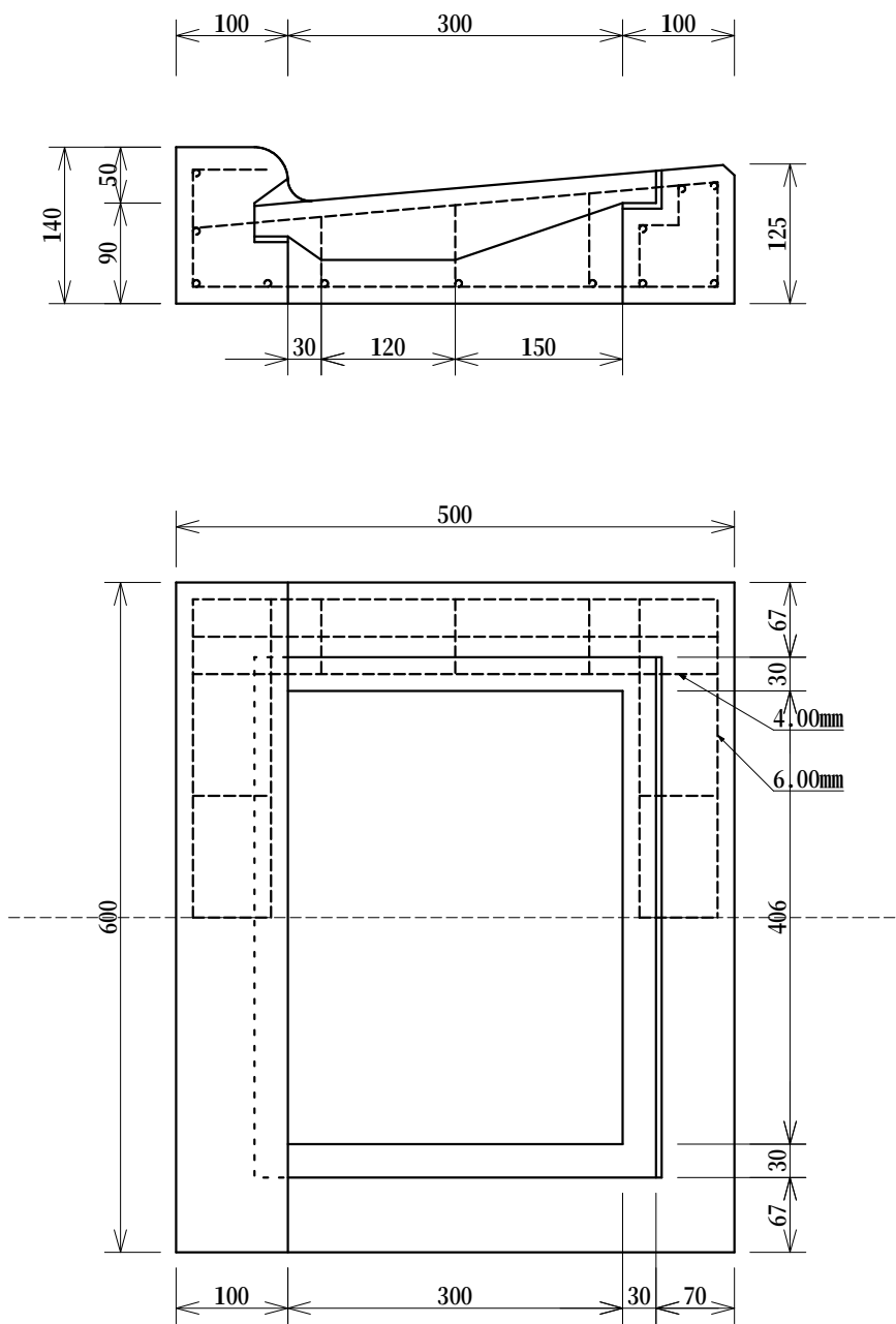
川崎市型雨水枡用平5cm縁塊 重量 約50kg
