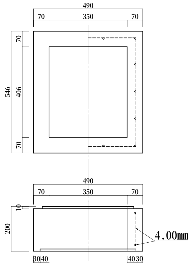
中部側塊 重量 約65kg
