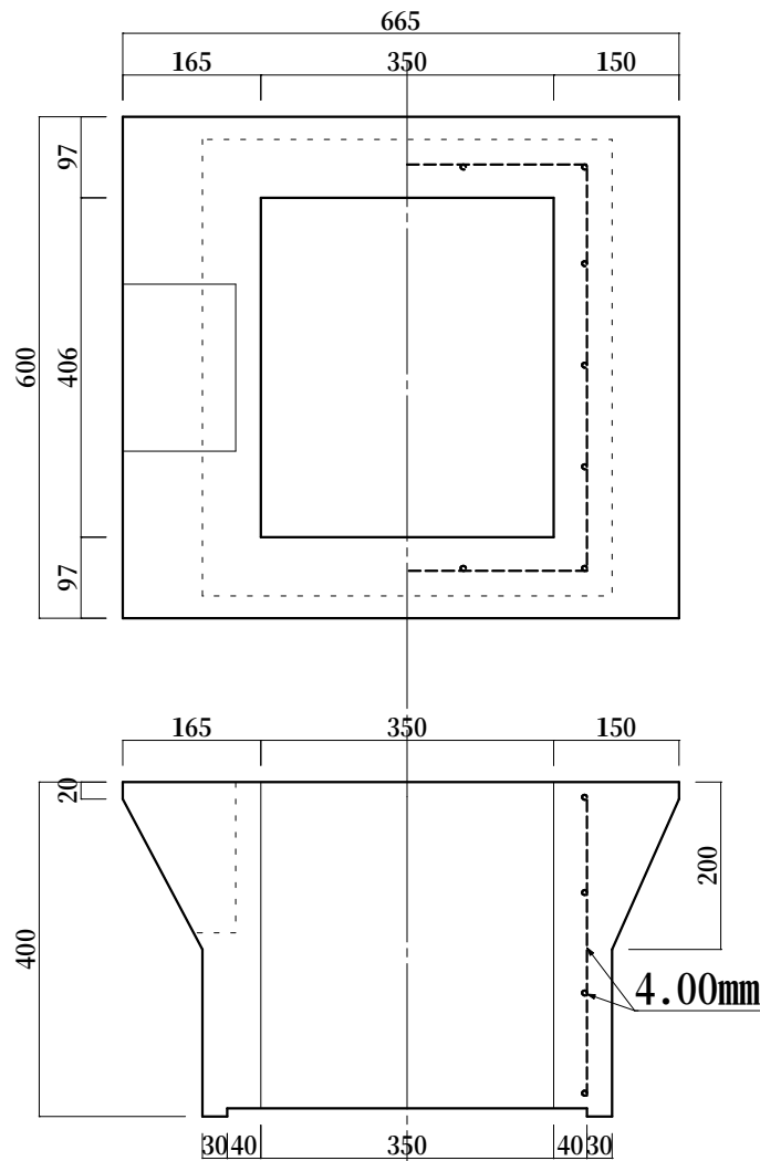
上部側塊 重量 約163kg
