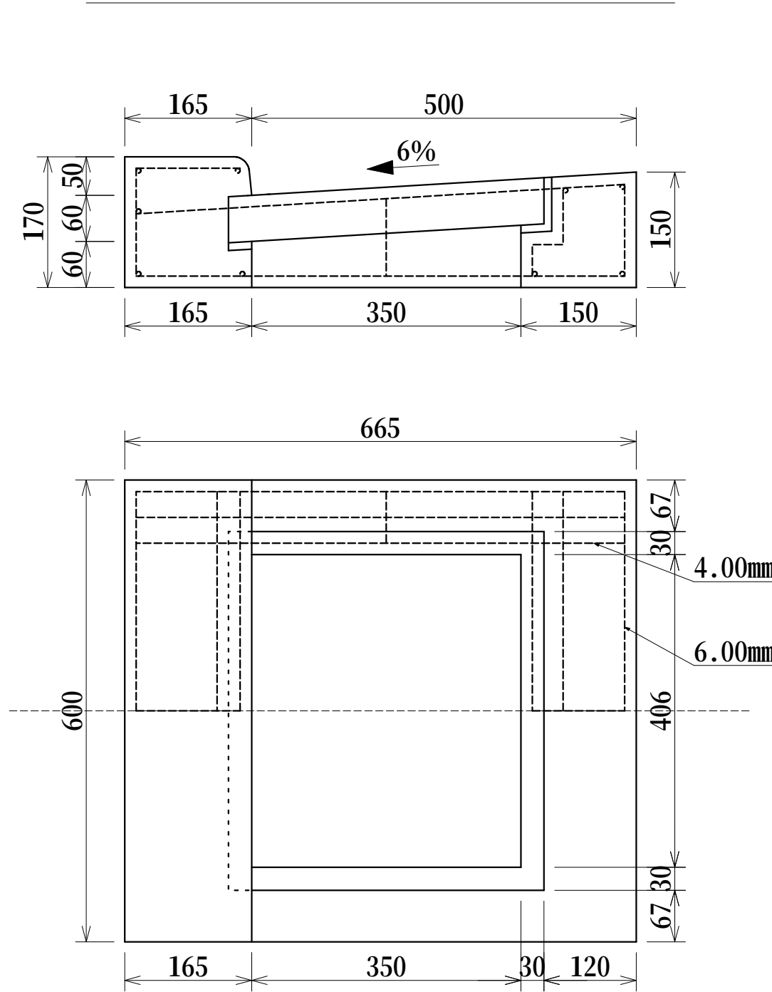
川崎市型街渠柵用平5cm縁塊 重量 約87kg
