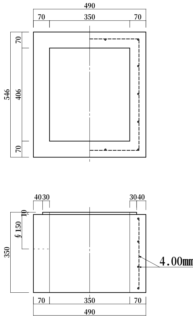
下部側塊 重量 約110kg
