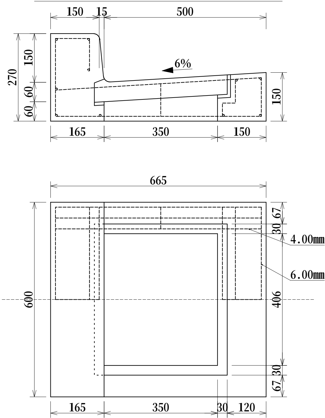
川崎市型街渠柵用真物縁塊 重量 約108kg
