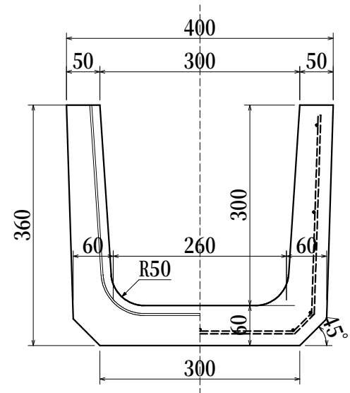
千葉県型長尺側溝 LDU 300×300×2000
