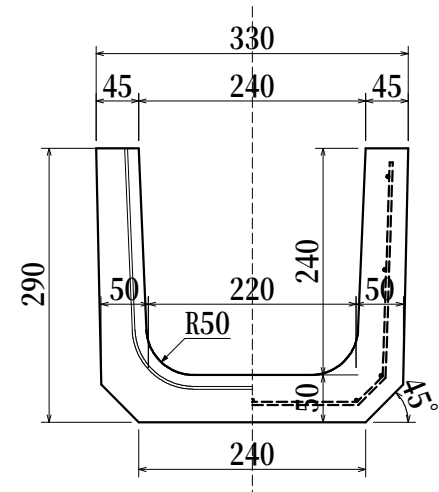
千葉県型長尺側溝 LDU 240×240×2000
