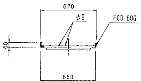
断面図
