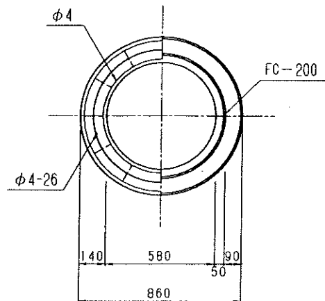
汚水蓋
