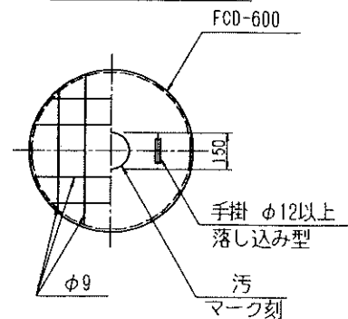
汚水蓋
