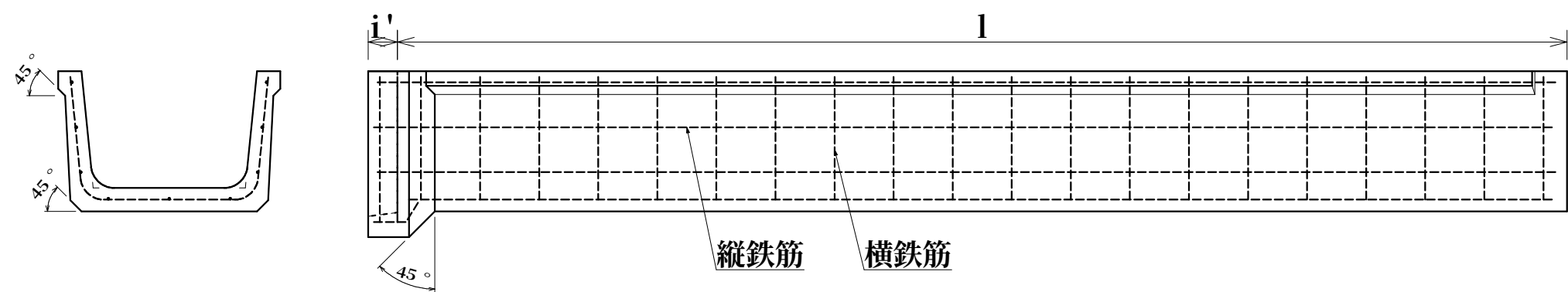
配筋図
