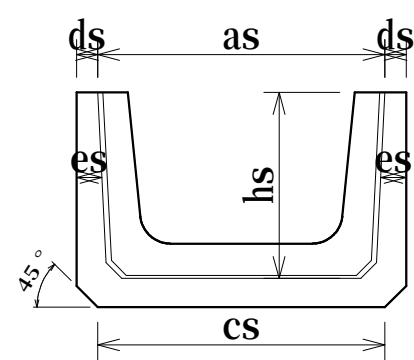
ソケット部
