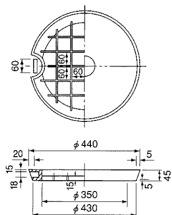
縁塊
