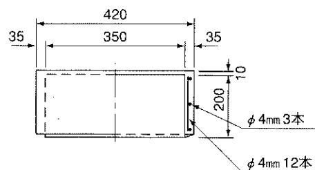
側塊高20cm
