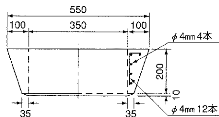
側塊異形乙
