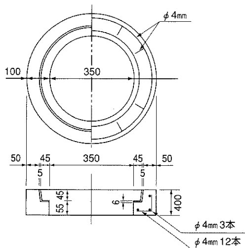
縁塊
