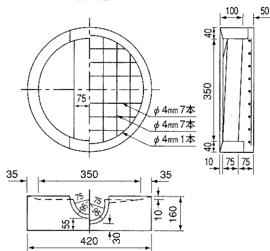
底版塊
