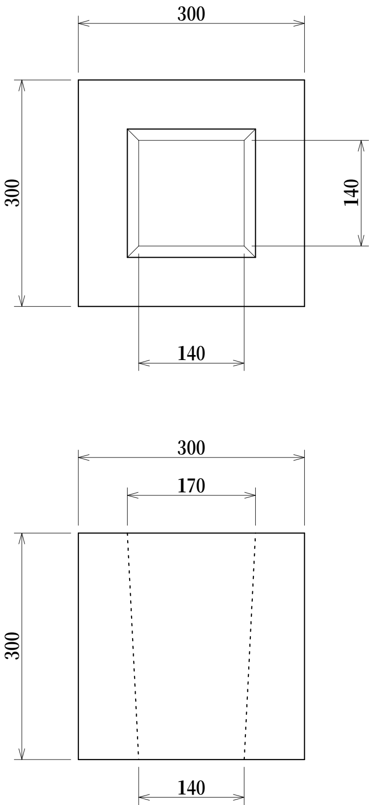
根固めブロック 300×300×H300 約49kg
