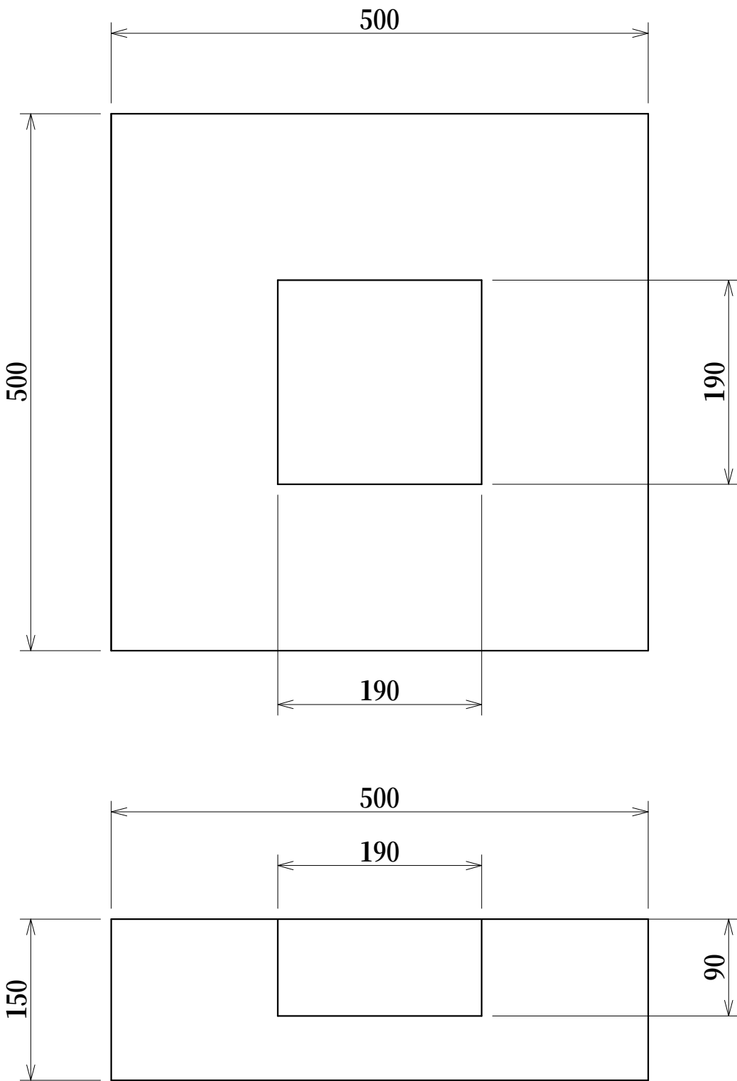
根固めブロック 500×500×150 (190×190×90) 約84kg
