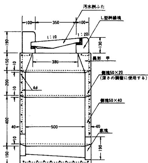
汚水枡（L型35cm用）
