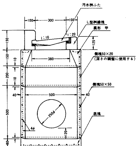
雨水枡（L型30cm用）
