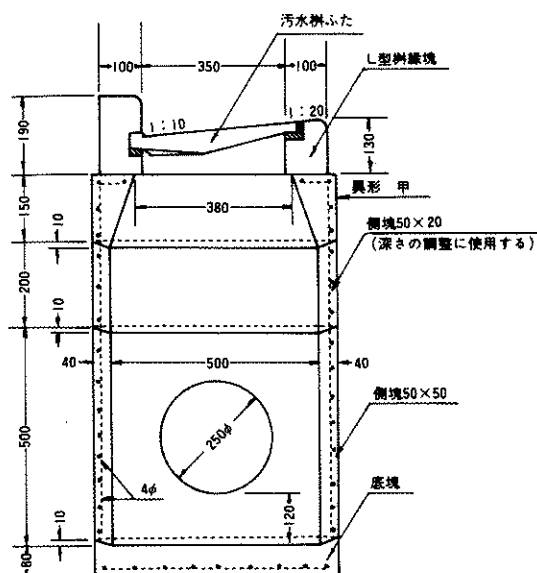
雨水枡（L型35cm用）
