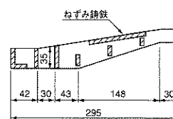
B-B断面
