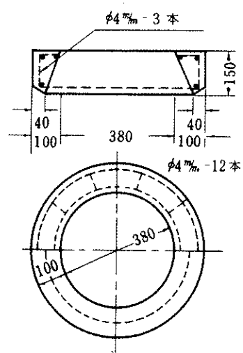
底塊50×9
