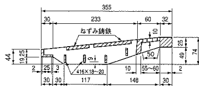
A-A断面
