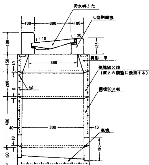
汚水枡（L型30cm用）
