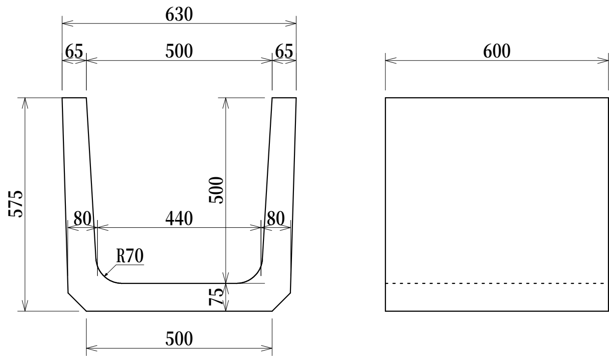
上ぶた式U形側溝本体 1種500（JIS規格外品）
