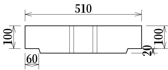
上ぶた式U形側溝ふた 2種400（JIS規格外品）
