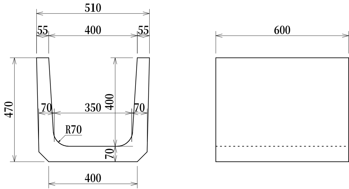
上ぶた式U形側溝本体 1種400B（JIS規格外品）
