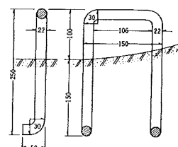
足掛金物
