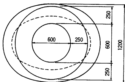
斜 壁
