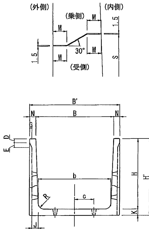
ジョイントテーパ部詳細図
