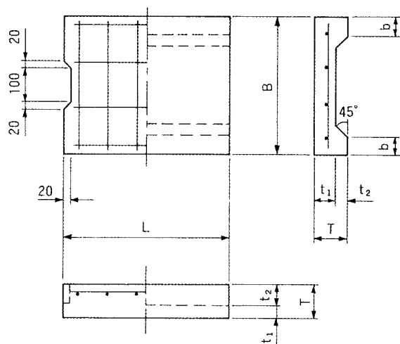
■PC3型歩道用
