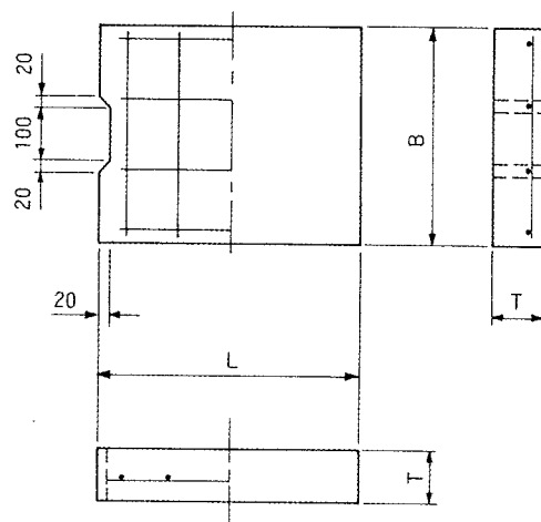
■PC4型車道用
