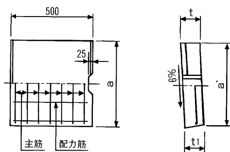
寸法表
