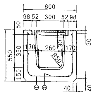
ストッパー部詳細
