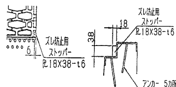
配筋
