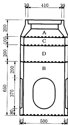
TMF-C (汚水)
