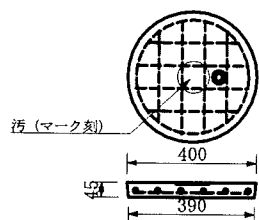
TMF-C (汚水)
