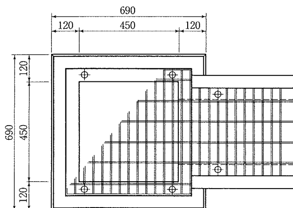
取付ます（240・300用）
