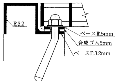
ボルト取付方法
