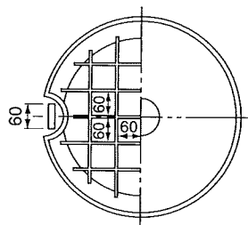
ふた
