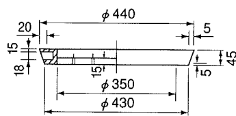
縁塊
