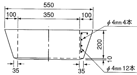
側塊異形乙
