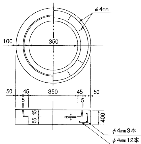
縁塊
