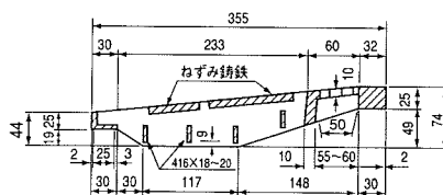
A-A断面
