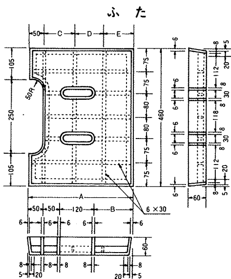
製品図
