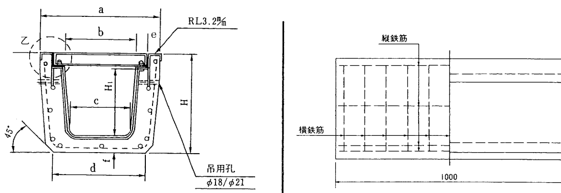
横断用U形 T-25（グレーチング固定式）
