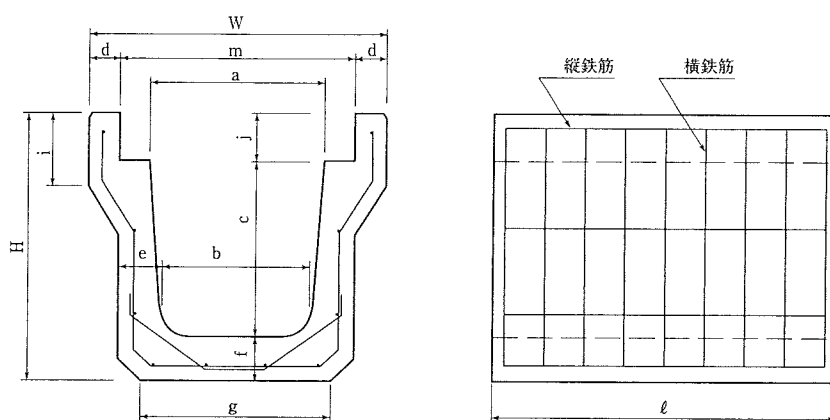
寸法表
