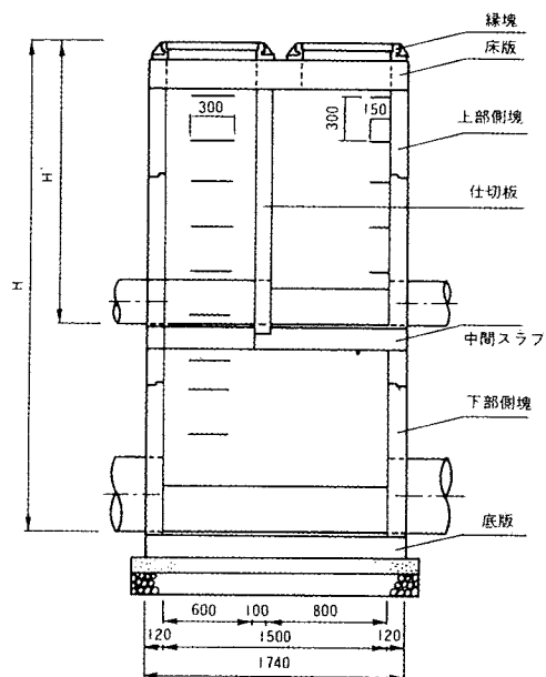
一般構造縦断面図
