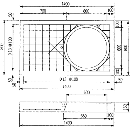
床版塊
