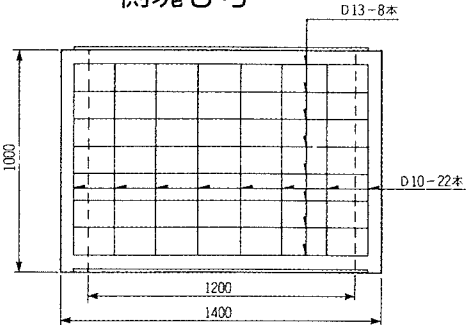
側塊 5 号
