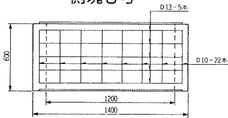
側塊 3 号
