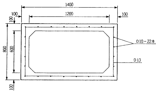
側塊 1 号
