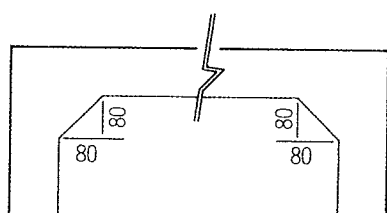
ハンチ詳細図
