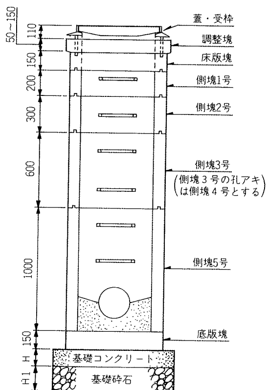
横断面図
