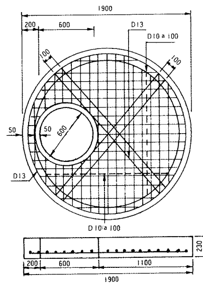
第3種 1900×230×600
