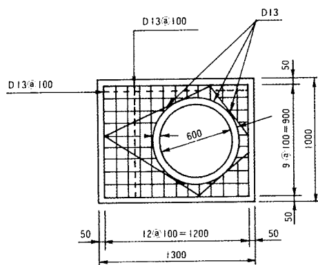
角型第1種 A型 1300×1000×600×200
